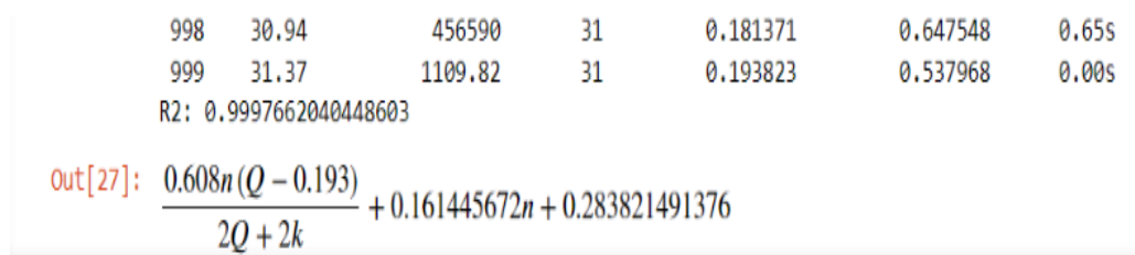
Рисунок 7 – Результат підбору формули нормуючого коефіцієнта відносно n, k при Q \in [0.1; 0.4]
